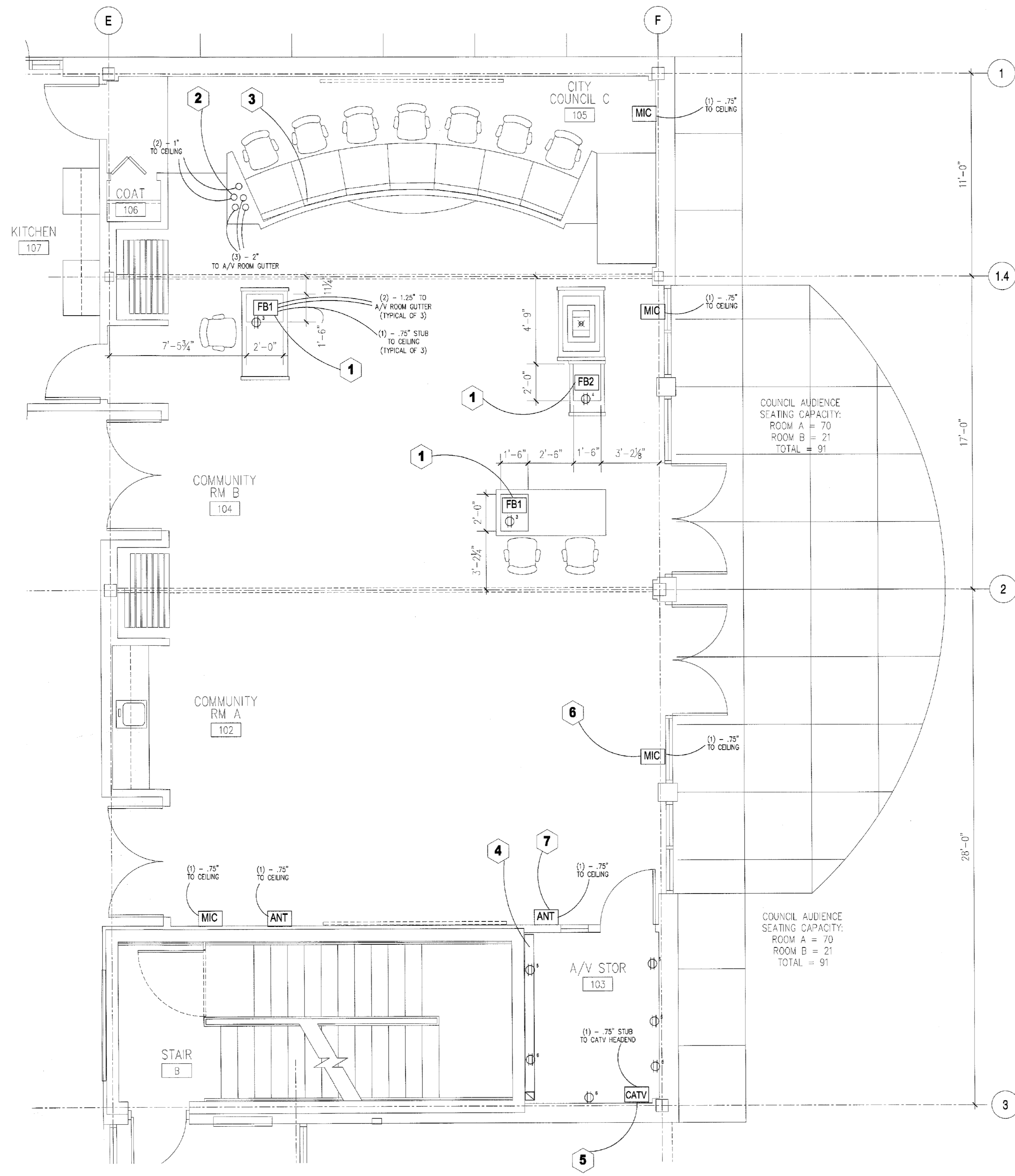
COUNCIL CHAMBERS AV FLOORPLAN
